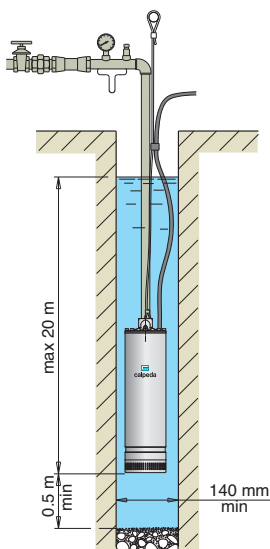
Pompa sospesa
